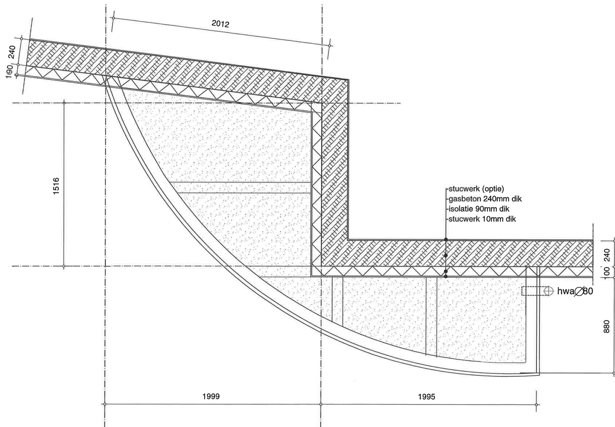
Bovenaanzicht luifel 1/10
