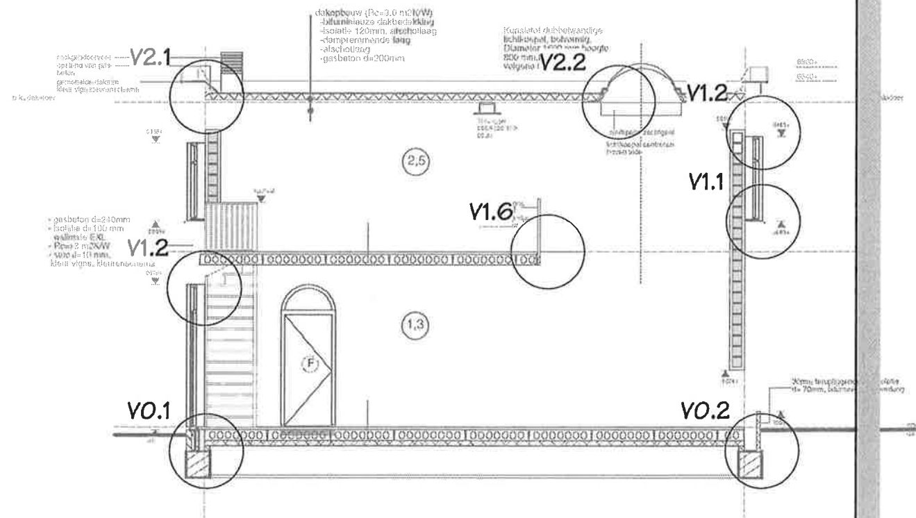
Type A: GEVEL TUIN WEST
